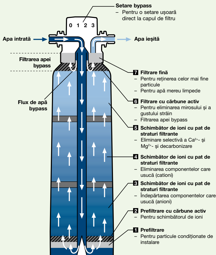
Structura unui cartuș filtrant BWT bestclear EXTRA cu filtrare cu 7 trepte
