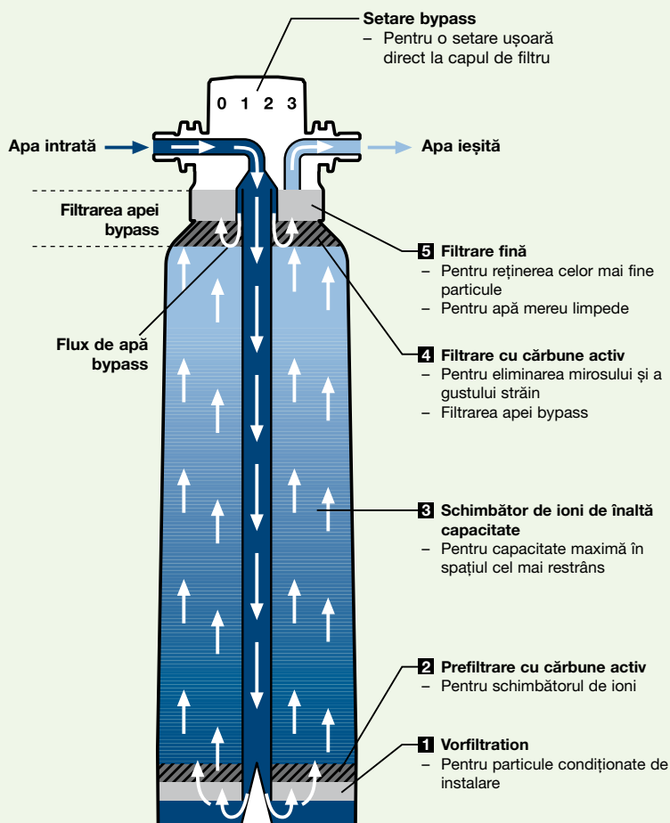
Structura unui cartuș filtrant BWT bestclear EXTRA cu filtrare cu 5 trepte
